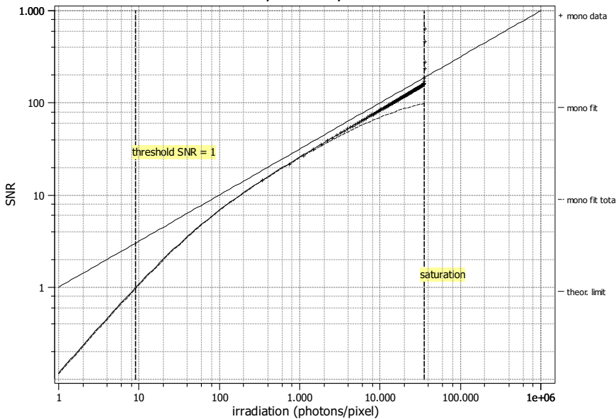
SNR m0801, 535 nm, 02.05.2019
